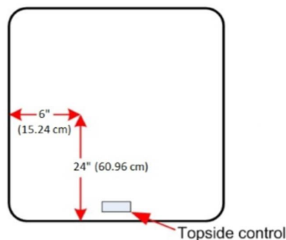
FIGURE 1: CONDUIT ÉLECTRIQUE EMLACEMENT
